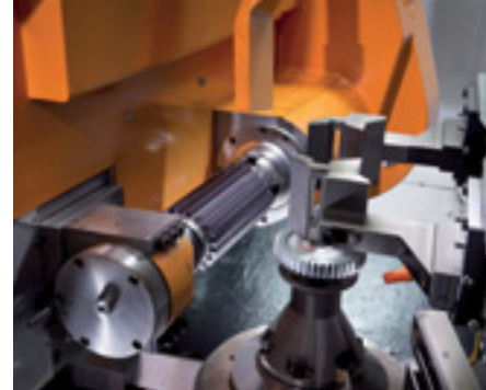
Machine de taillage robotisée, production d'engrenages
